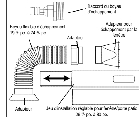
Fig. 1 Accessoires d'installation
